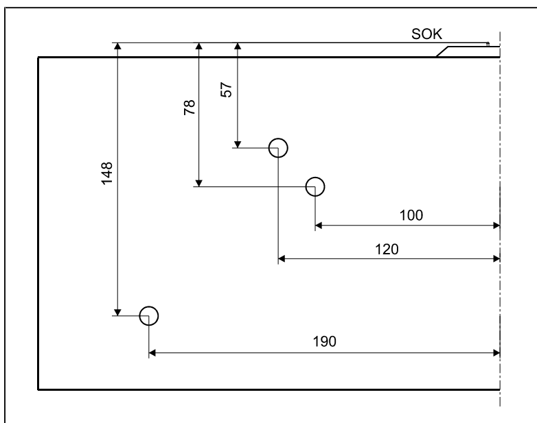
Abbildung 2: Anordnung der Bohrungen in Bezug auf die Gleisachse und die Schienenoberkante
