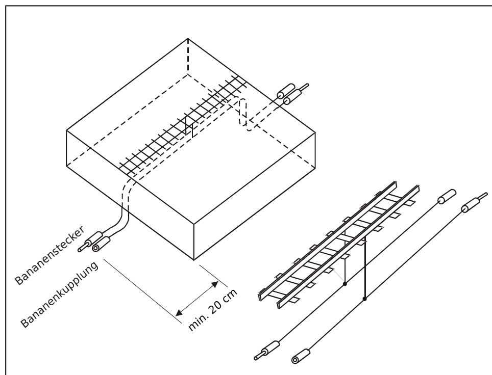
Abbildung 1: Verkabelung eines Moduls
